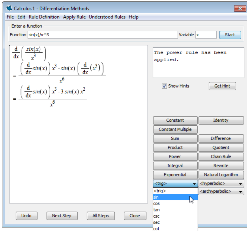
図5.11 微積分 1 - 微分法チューター
