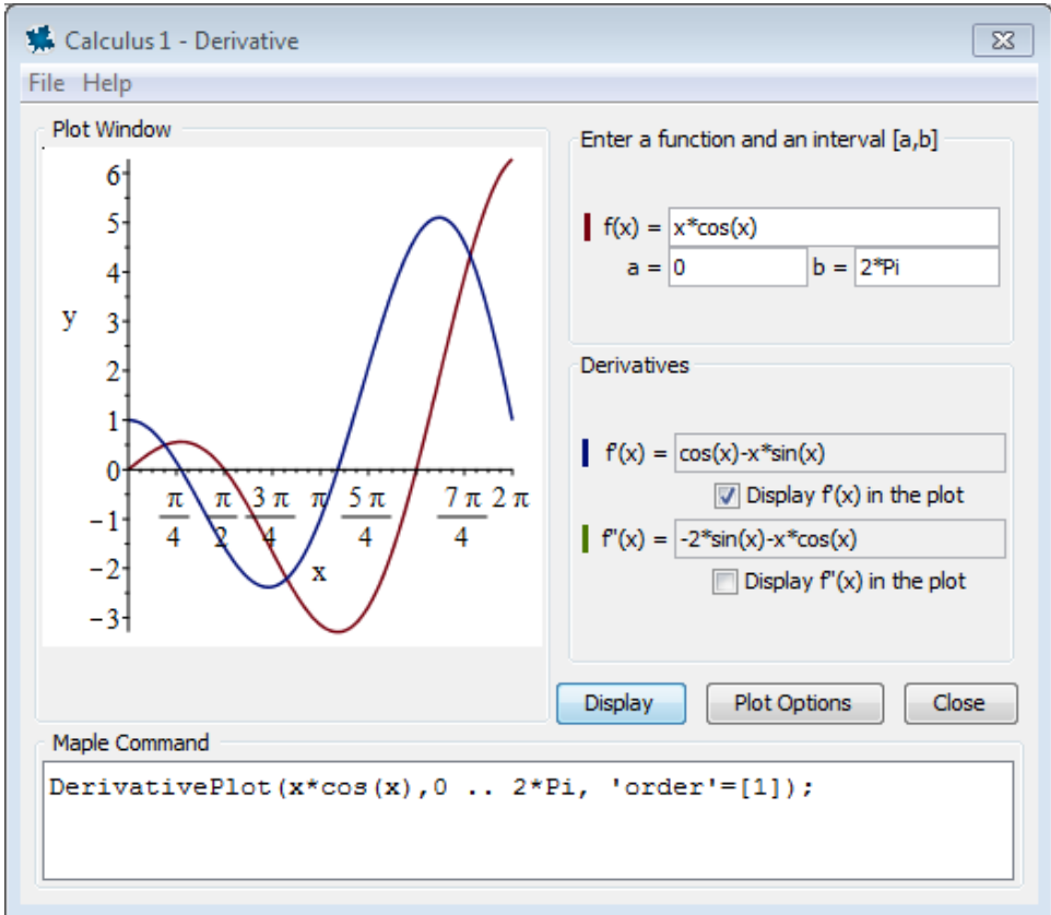
図5.10 微積分 1 - 微分チューター
