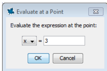
図8.2 点で評価
