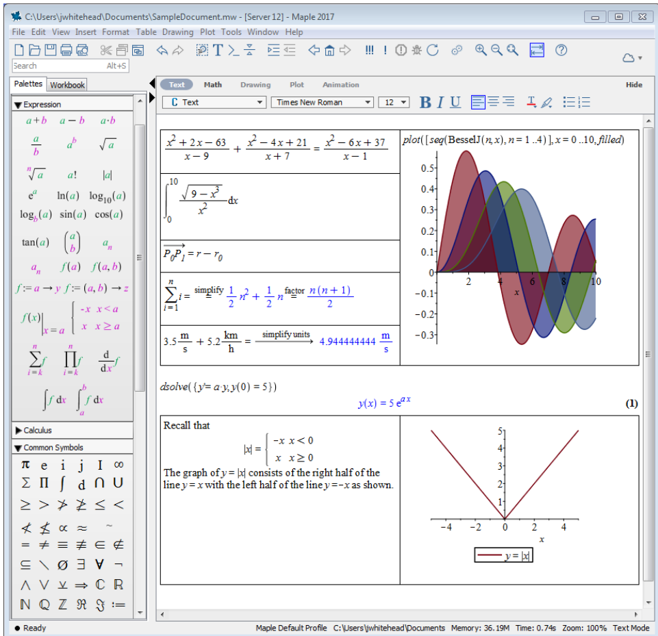
図1.1 Maple 環境
