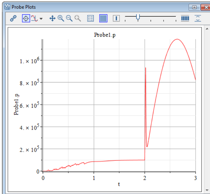
図6.31 アクムレータを持つ場合の圧力サージ
