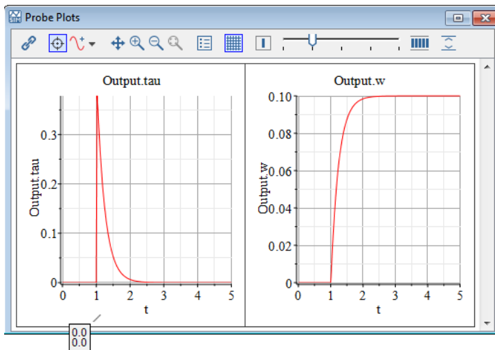
図1.10 DC Motor のトルクとスピードのプロット
