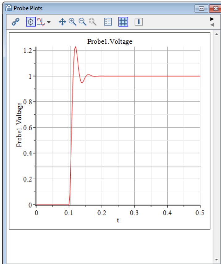
図1.8 電圧レスポンスのプロット
