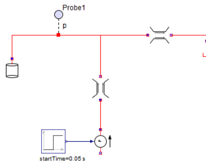
図6.24 油圧作動油の圧縮率
