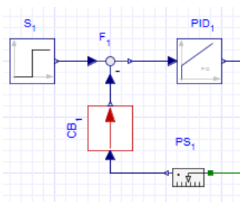
図2.5 Conversion Block を使用した単位の指定
