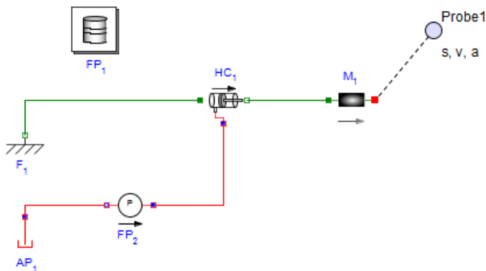
図6.19 固定圧力源を使用した並進運動
