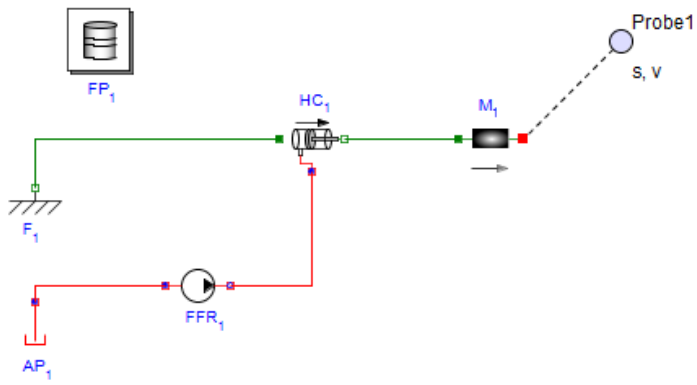
図6.18 固定流量源
