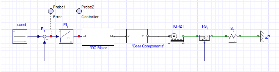
図6.1 ケーブル張力コントローラ
