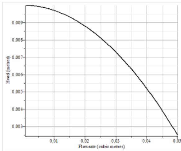
図6.11 遠心ポンプの水頭流量曲線
